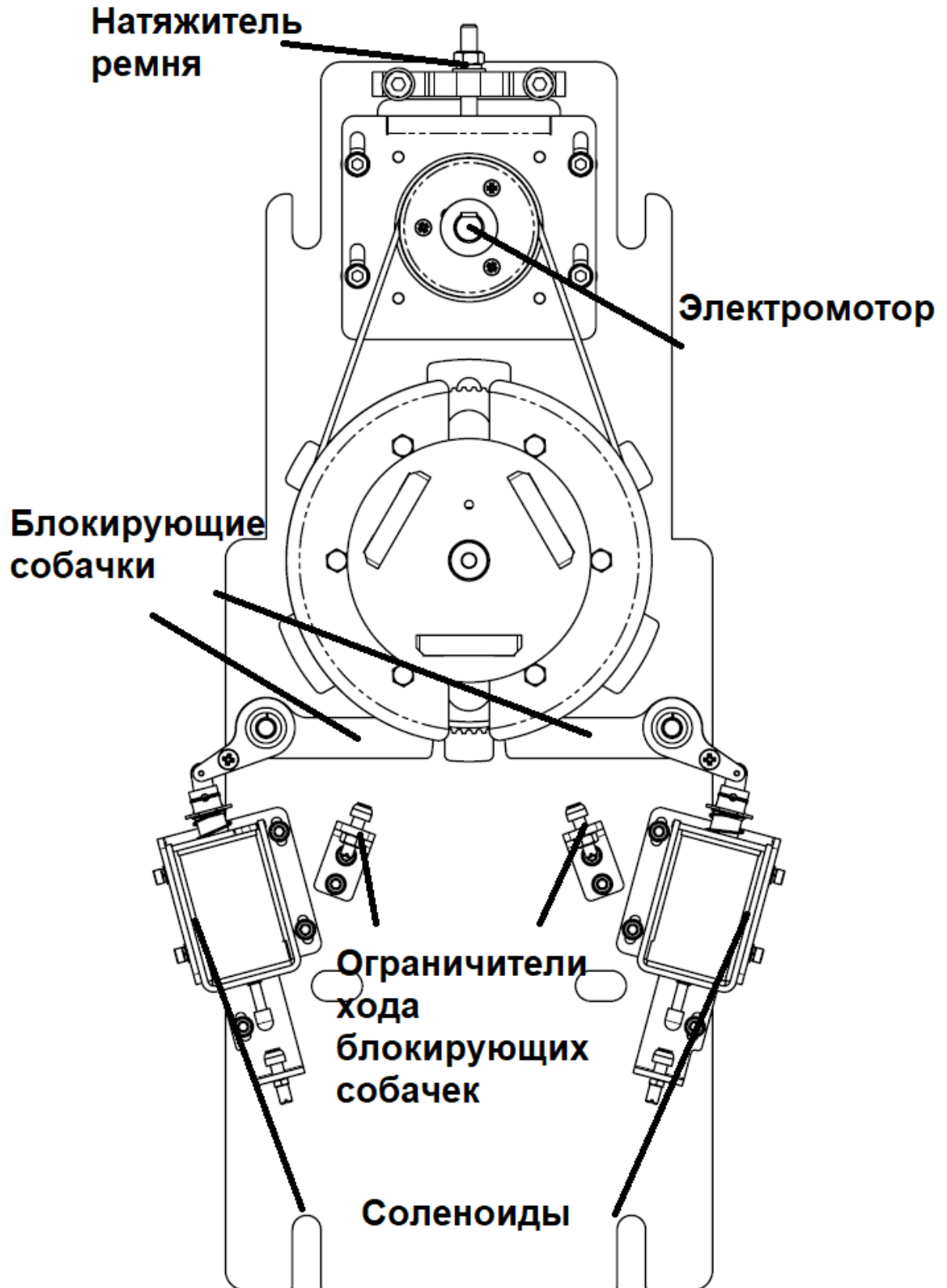
Рисунок 5 – Внешний вид
